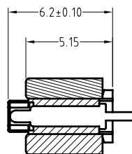
剖面 B-B
