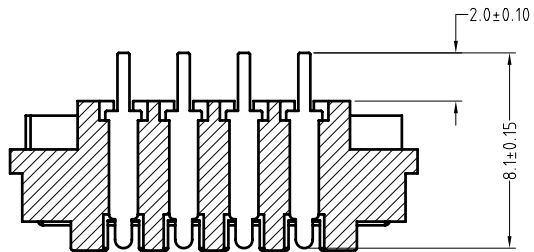
剖面 A-A
