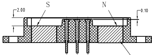
剖面 A-A
