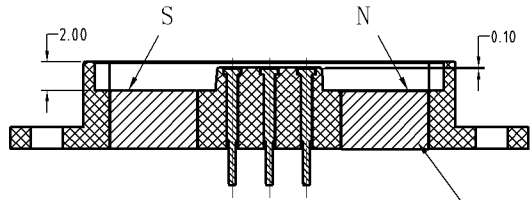
剖面 A-A
