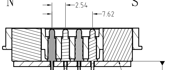
截面 A-A
